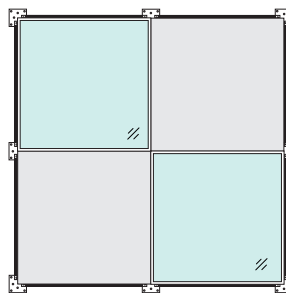
Sistema de suelo técnico con baldosa GAMAFLOR GLASS incorporada
