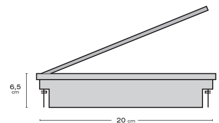
Boîte électrique ouverte
